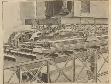
Fig. 2. — Detalle del mecanismo. — P. Patín de los wagones. — R. Rail de desahorro. — A. Alabes del wagon que reciben el chorro de agua de propulsión. — B. Extremo del propulsor por donde sale el agua. — D. Amortiguador. — C. Cadenas colgantes sin fin.
